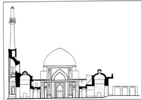
یزد، مسجد جامع، برش و نما ( ژوینر ) .
