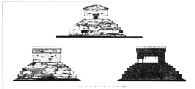
پاسارگاد، طرحی قدیمی از آرامگاه کوروش. پاسارگاد، برش و نما از آرامگاه کوروش (از کتاب مجموعه اثر معماری سستی ایران).
