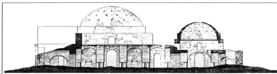
کاخ سروستان، برش از اتاق کعبه دار کوچک (از مجموعه آثار معماری سنی ایران).
