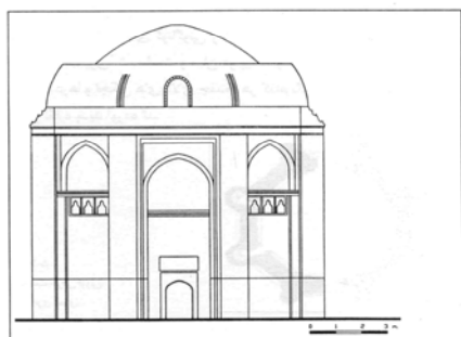
برج خرقان قزوین، ۴۶۰ هجری قبری، برش یکی از قدیمی ترین گنبد های گسسته در جهان.
