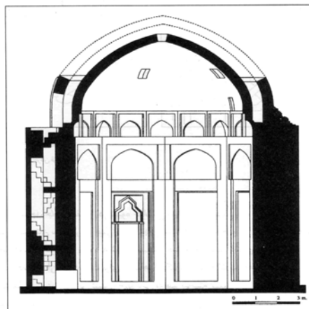
برج دوم خرقان قزوین، ۲۸۶ هجری قمری، برش
