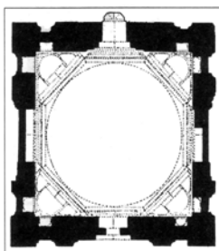
دوارة نام برد - ۴۰ هجری قمری (رنگش شده بود).
