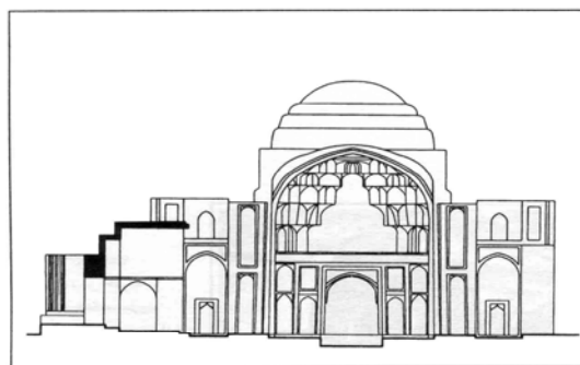
مسجد جامع ورامین، نقشه کنونی. مسجد جامع ورامین، نما - برش (از مرکز اسناد نقشه معماری و شهرسازی دانشگاه علم و صنعت ایران). مسجد جامع ورامین، طرحی از درون رواق ها (از مامد دیولوا).
