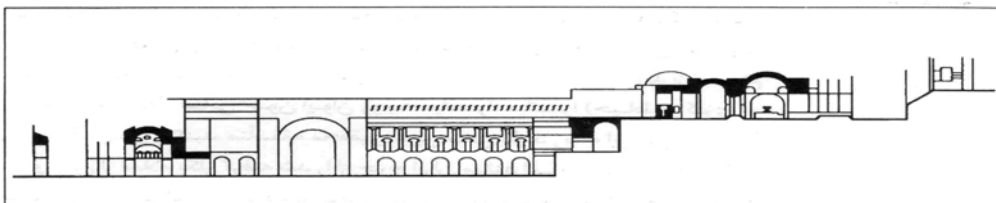
ارسن کوه خواجه، برش طولی (از کتاب میراثوری پارتها)
